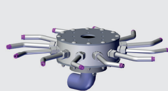
Streueinheit BrineStar
